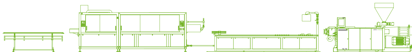
采用双螺杆挤出机的型材挤出生产线
